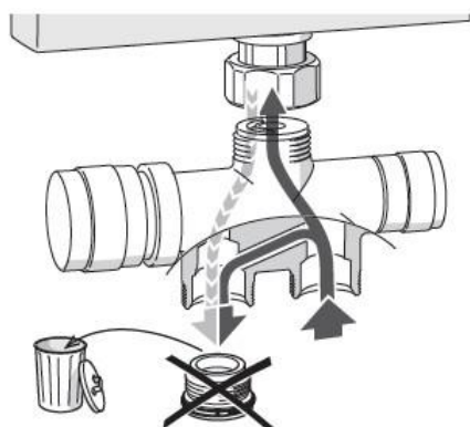
Standartní verze (ONE PIPE SYSTEM)
